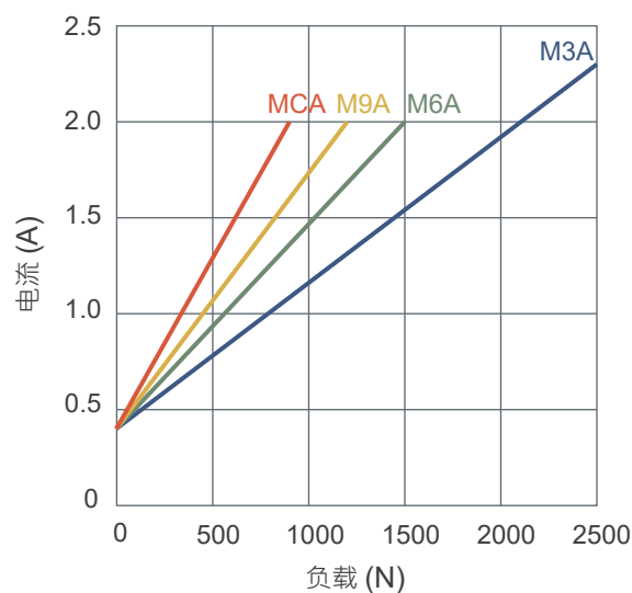
电流 VS. 负载
