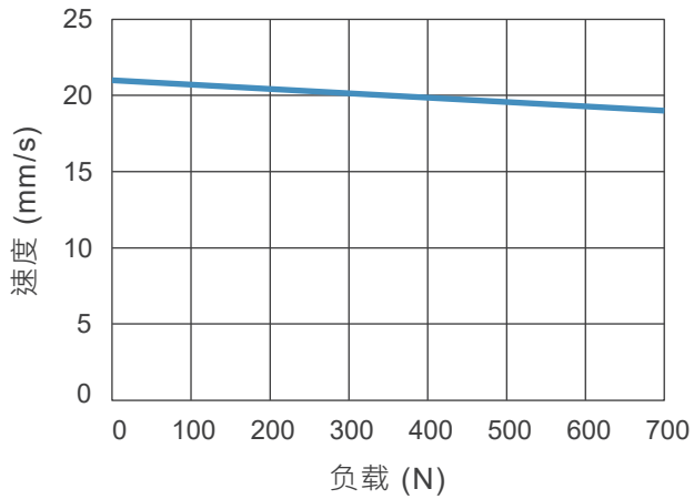
速度 VS. 负载
