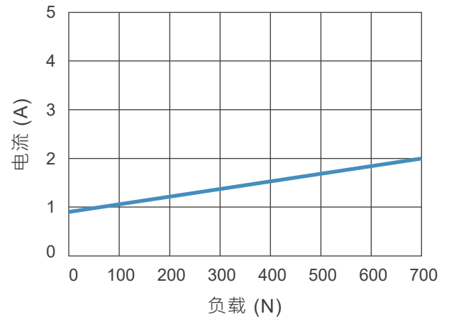
电流 VS. 负载
