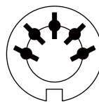
5-pin DIN socket
