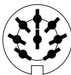
8-pin DIN socket
