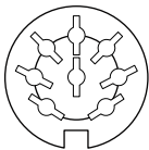
8-pin插座
