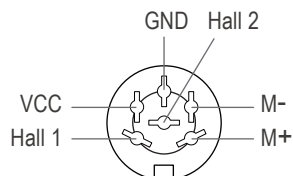
6-pin 插座
